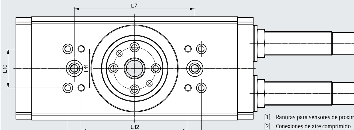
DRRD-50/63
