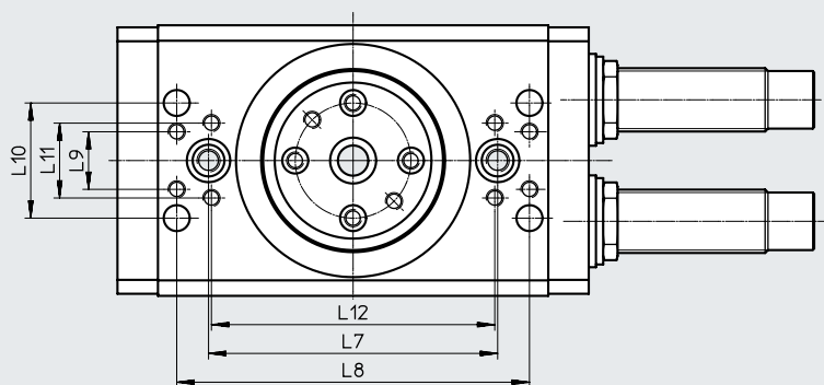
DRRD-32 ... -40
