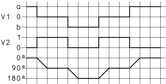
Secuencia del control
