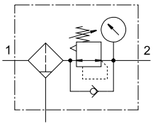
Kondensatablass halbautomatisch, mit Manometer
