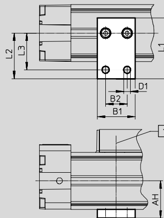
Ø 18/25 s MUP-18/25-P (na jednostrannú montáž)
