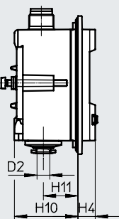
SPAU-...-F-Q-...-D-...-MxU SPAU-...-F-T532D-...-MxU
