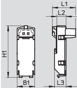
전기 연결 플레이트, S2/H2
