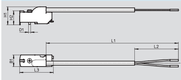
전기 연결 플레이트, VK6 ... 9
