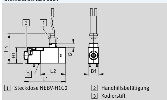
Steckeranschluss oben
