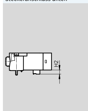
Steckeranschluss unten
