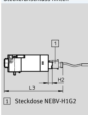
Steckeranschluss hinten
