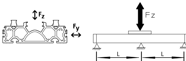
Kraft Fz
