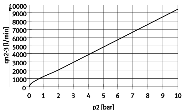
Durchfluss q_n von 2 \rightarrow 3 in Abhängigkeit vom Ausgangsdruck p_2 VPPX-12L-...-0L10H-... (10 bar)
