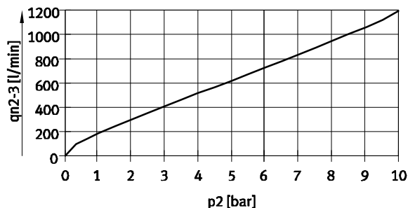
Durchfluss q_n von 2 \rightarrow 3 in Abhängigkeit vom Ausgangsdruck p_2 VPPX-6L/F-...-0L10H-... (10 bar)
