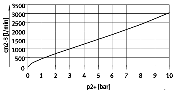
Durchfluss q_n von 2 \rightarrow 3 in Abhängigkeit vom Ausgangsdruck p_2 VPPX-8L-...-0L10H-... (10 bar)
