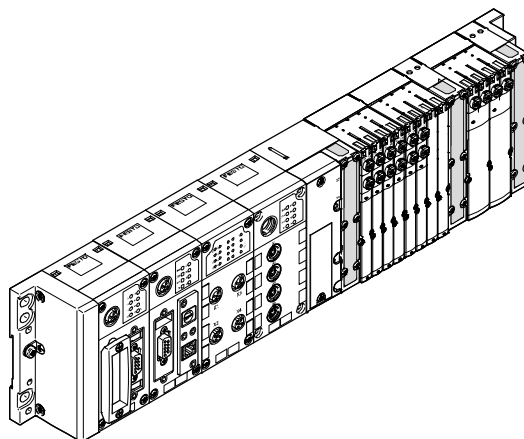
in Metallausführung mit Ventilinsel VTSA – zentral
