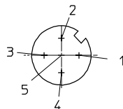
1 Conector tipo clavija M12x1, 5 contactos
