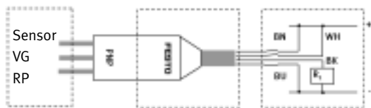
Kabelbaum zur VADMI
