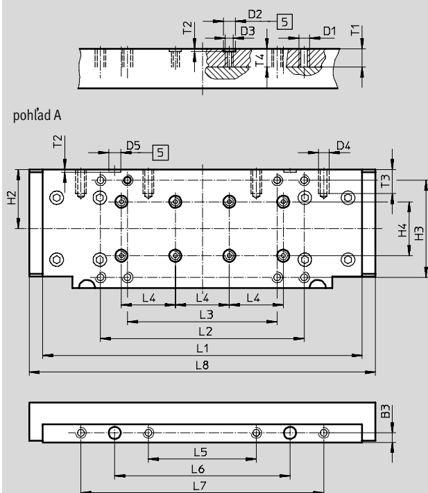
pohľad A
