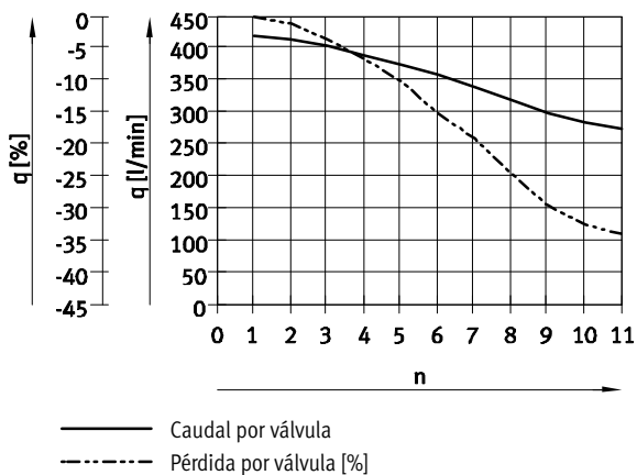
Caudal q por válvula, al activarse simultáneamente varias (n) válvulas (tolerancia ± 20%)
