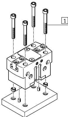
1 Befestigungsschrauben 2 Zentrierstifte, Zentrierhülsen
