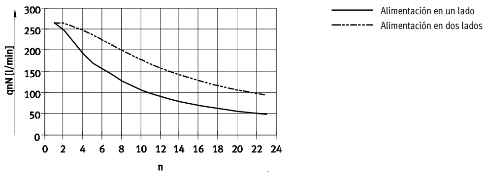
Caudal nominal normal q_{pN} con válvulas de 5/2 vías con varias válvulas n conmutadas simultáneamente, tamaño 10
