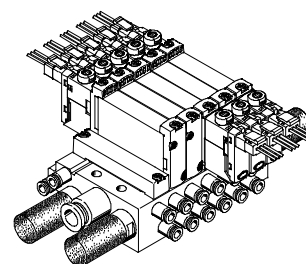
Batería de válvulas VTUG compuesta por válvulas para placas base VUVG-B
