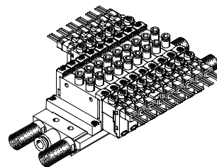
Batería de válvulas VTUG compuesta por válvulas con conexiones roscadas VUVG-S
