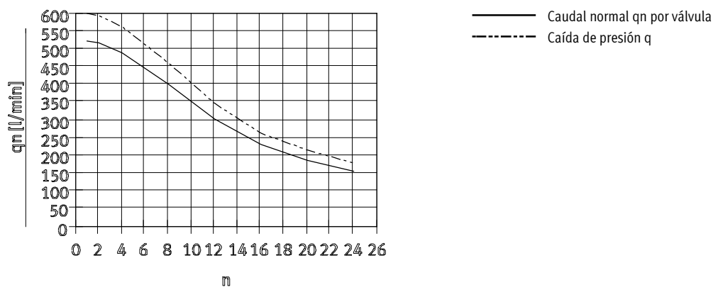
Caudal normal q_n en función de la cantidad de válvulas n conmutadas, tamaño 14
