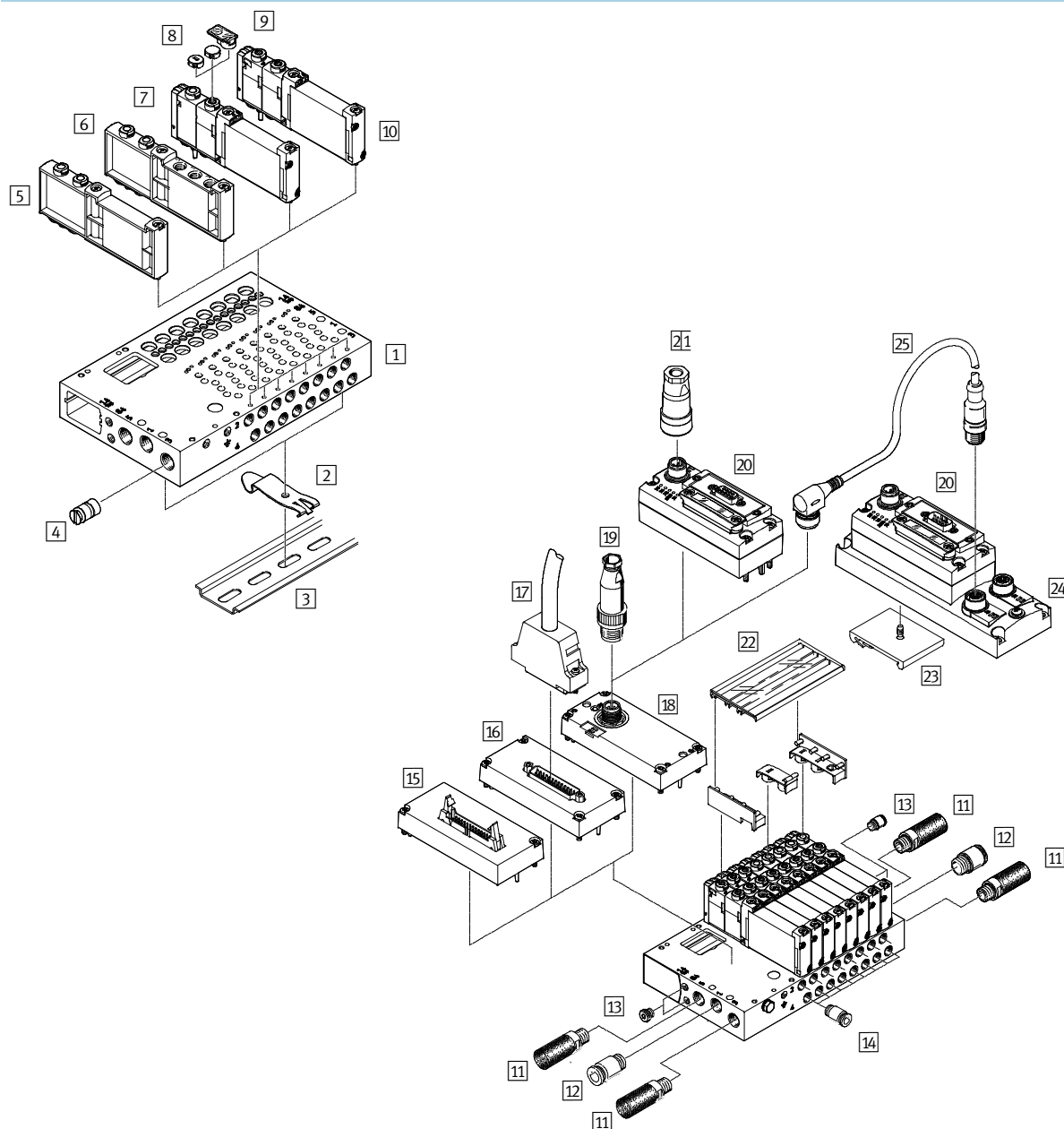
Cuadro general de terminal de válvulas. Válvulas para placas base
