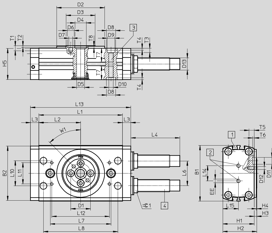
DRRD-...-P
