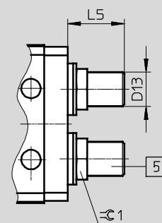
DRRD-...-P
