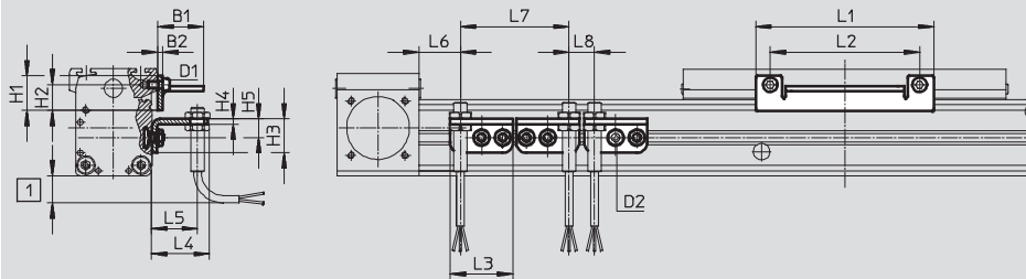
DGE-25-...-ZR-RF-...
