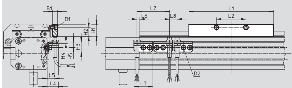
DGE-40/-63-...-ZR-KF-...
