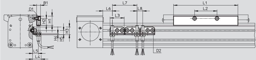
DGE-40/-63-...-ZR-RF-...
