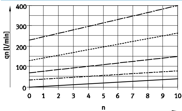
Caudal nominal normal qn con 6 bar → 0 bar en función de la posición del tornillo de estrangulación (escala) n
