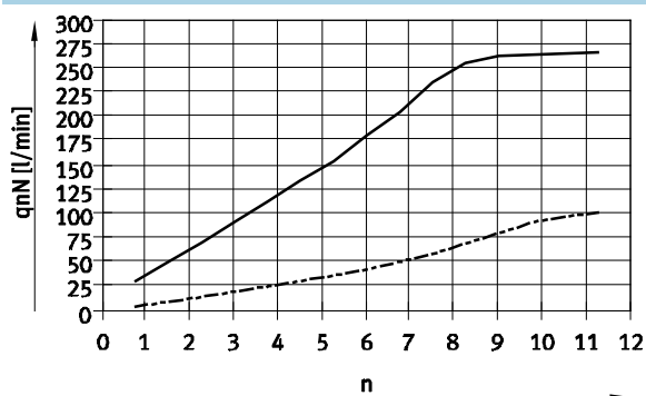
Caudal nominal normal q N con 6 → 5 bar en función de los giros n del husillo
