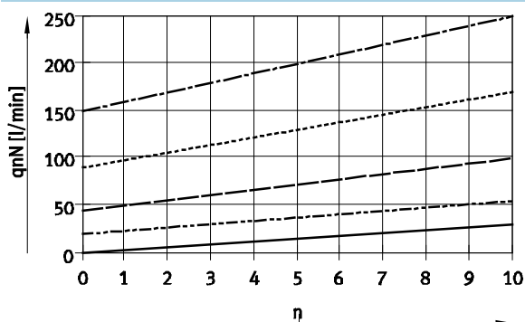
Caudal nominal normal qnN con 6 bar → 5 bar en función de la posición del tornillo de estrangulación (escala) n
