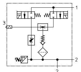
avec impulsion d'éjection et vacuostat
