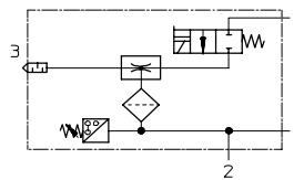
VADM-...-P/-N avec vacuostat
