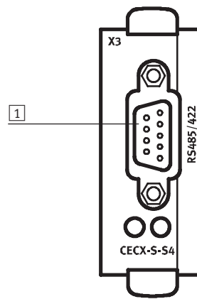
1 RS 485-A/422-A-Anschluss
