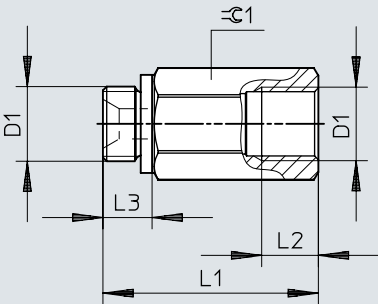
Dimensiones – H-1/8-A/I
