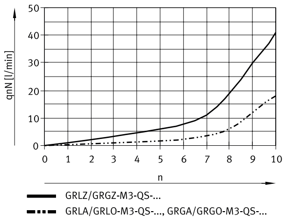
Normalnennendurchfluss q_{nN} bei 6 → 5 bar in Abhängigkeit der Spindelumdrehungen n (GRLA/GRLZ-M3, Mini – Steckanschluss QS, Metall)
