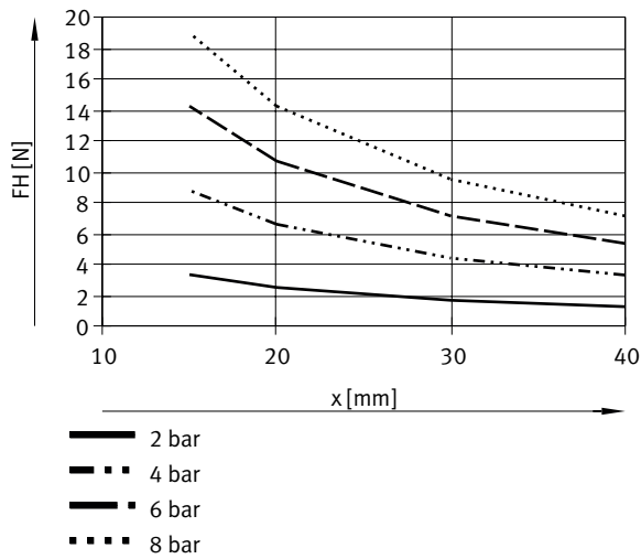
Greifkraft FH pro Greifbacken in Abhängigkeit vom Betriebsdruck und dem Hebelarm x – Innengreifen (öffnen), doppelwirkend – DHWS-10
