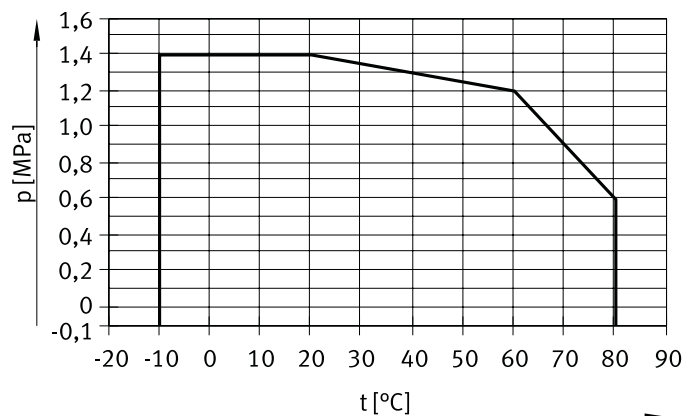
工作压力 p 与温度 t 的关系 (QS-G3/4-22 除外)
