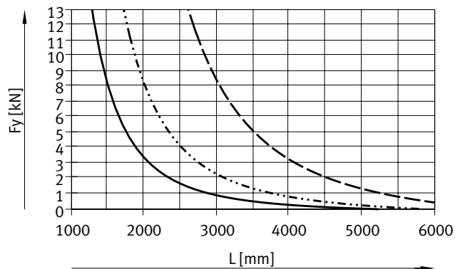
力 F_y
