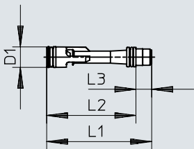
Dimensions – VN-07/10
