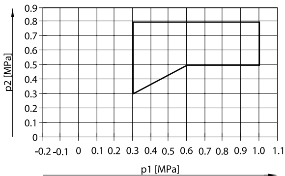
[1] 外部パイロット給気の場合のメインバルブ使用圧力範囲
