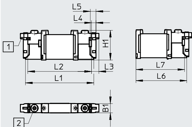
[1] Elektrischer Anschluss vertikal [2] Handhilfsbetätigung
