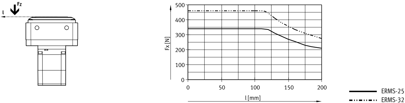
最大动态径向力 F z 与杠杆臂的关系 l
