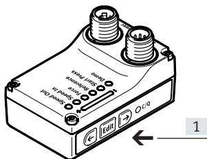
[1] tlačidlá na parametrizáciu a ovládanie
