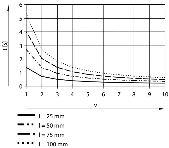
Polohovací čas t v závislosti od rychlosti v a zdvíhu l s paralelnou kostrukčnou súpravou pre EGSS-BS-32
