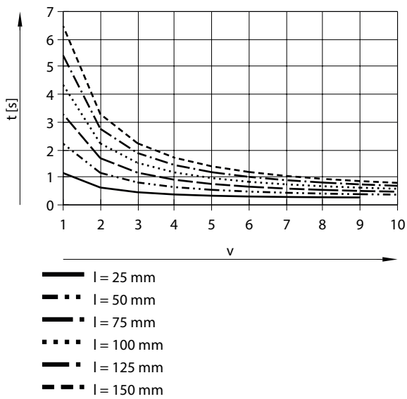
Polohovací čas t v závislosti od rychlosti v a zdvíhu l s paralelnou kostrukčnou súpravou pre EGSS-BS-45
