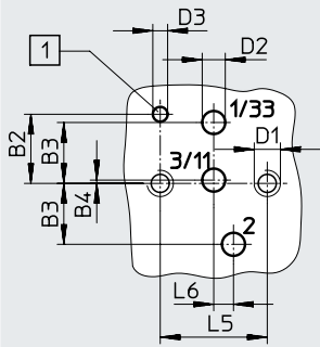
[1] Taladro para codificador
