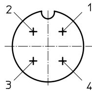
[1] Anschluss-Stecker M12x1, Stift, 4-polig nach EN 61076-2-101
