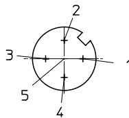
[1] Anschlussstecker M12x1, Stift, 5-polig
