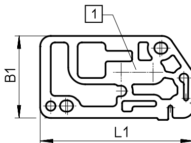
[1] ohne Langloch, Steuerluftversorgung extern
