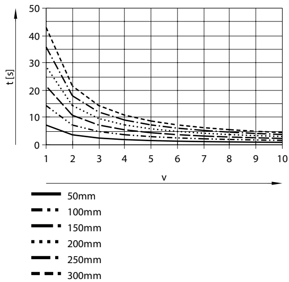
Positionierzeit t in Abhängigkeit von Geschwindigkeitsstufe v und Hub l mit Parallelbausatz für EPCS-BS-45-3P
