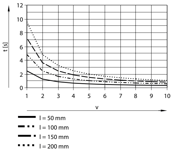
Positionierzeit t in Abhängigkeit von Geschwindigkeitsstufe v und Hub l mit Axialbausatz für EPCS-BS-32-8P
