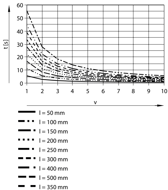
Positionierzeit t in Abhängigkeit von Geschwindigkeitsstufe v und Hub l mit Axialbausatz für EPCS-BS-60-5P
