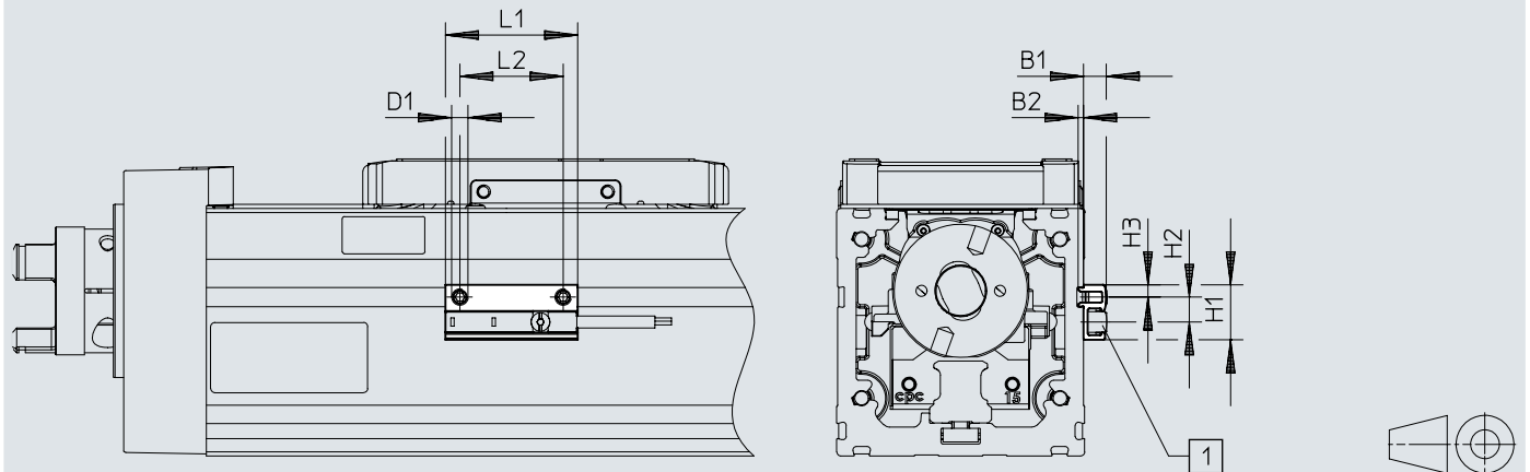
[1] Näherungsschalter
