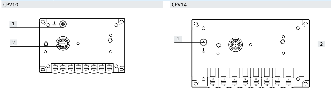
[1] Erdungsschraube [2] I-Port Schnittstelle/IO-Link [1] Erdungsschraube [2] I-Port Schnittstelle/IO-Link
