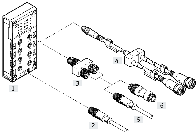
Kombination Anschlussblock mit elektrischer Verbindungstechnik
