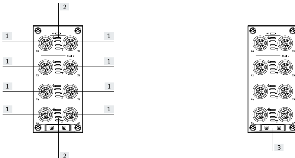
[1] Elektrischer Anschluss Eingänge [2] LED-Anzeigen
