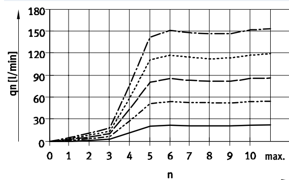
Normálny prietok q_n [l/min] v závislosti od otáčok skrutky n VFFK-C-K-M5-P VFFK-C-K-M7-P
