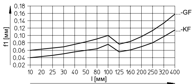
DFM с 2 подшипниками на направляющий стержень
