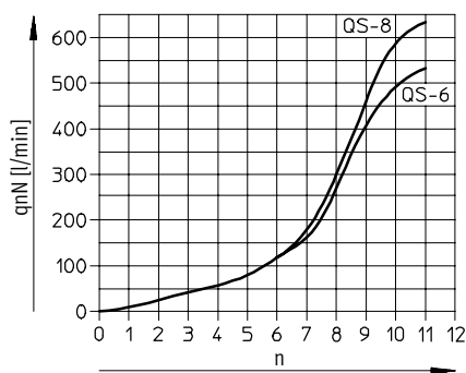
Portata nominale normale qnN a 6 bar → 5 bar in funzione del numero di giri della vite n Filettatura G1/8, G1/4, G3/8
