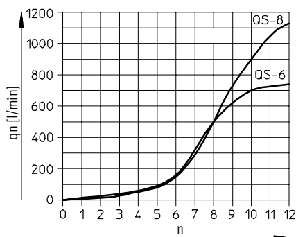
Portata normale qn a 6 bar → 0 bar in funzione del numero di giri della vite n Filettatura G1/8, G1/4, G3/8
