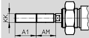
K2 – Stelo con filetto maschio prolungato
