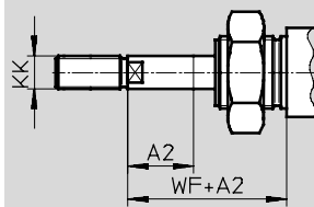
K8 – Stelo prolungato
