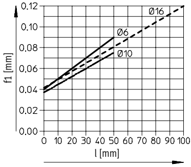
Tige de piston traversante avec guidage à palier lisse GF
