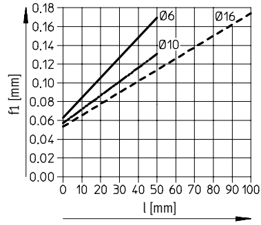
Tige de piston traversante avec guidage par recirculation de billes KF
