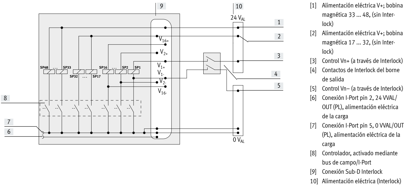
Ejemplo de esquema del circuito de la interfaz Interlock de dos pines
