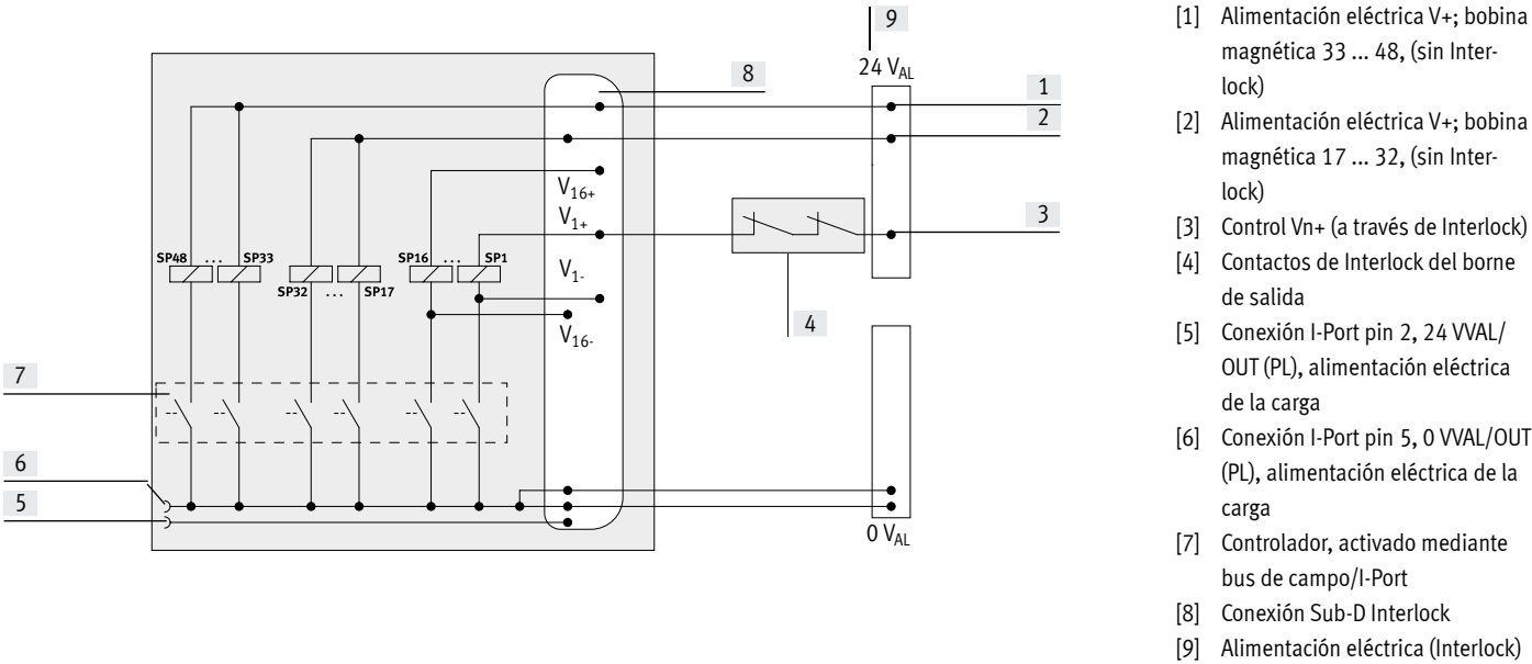
Ejemplo de esquema del circuito de la interfaz Interlock de un pin
