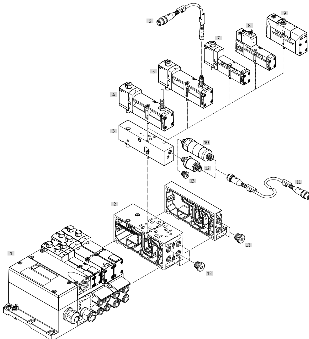
Cuadro general de periféricos de la válvula de conmutación del aire de pilotaje
