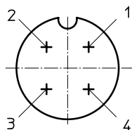
[1] Conector M12x1, pasador, 4 pines según EN 61076-2-101
