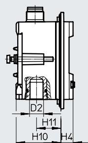
SPAU-...-F-Q...-Mx SPAU-...-F-T532...-Mx
