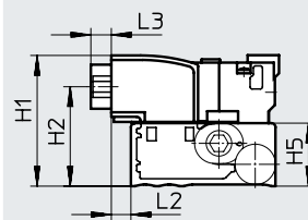
Salida del conector hacia el lado eléctrico
