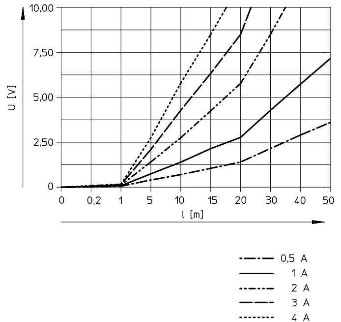
Caída de tensión U con sección de cable de 0,25 mm 2 con M12
