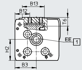
∅ 18 ... 40
