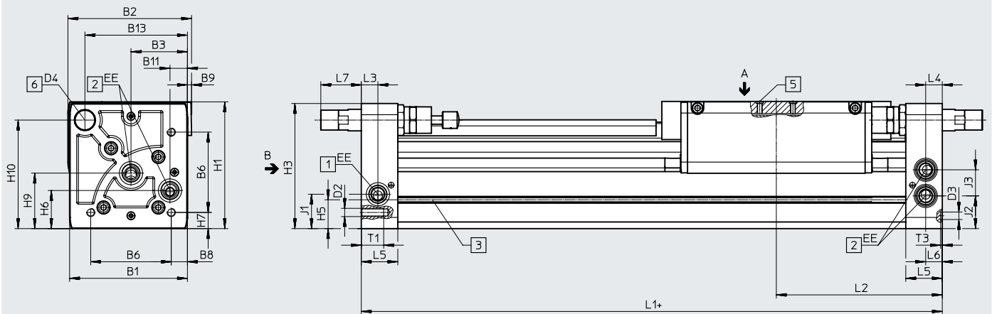
∅ 50 Ansicht B ∅ 50 ... 63
