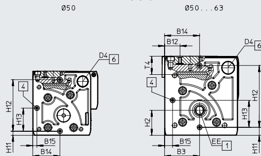
Ansicht B
