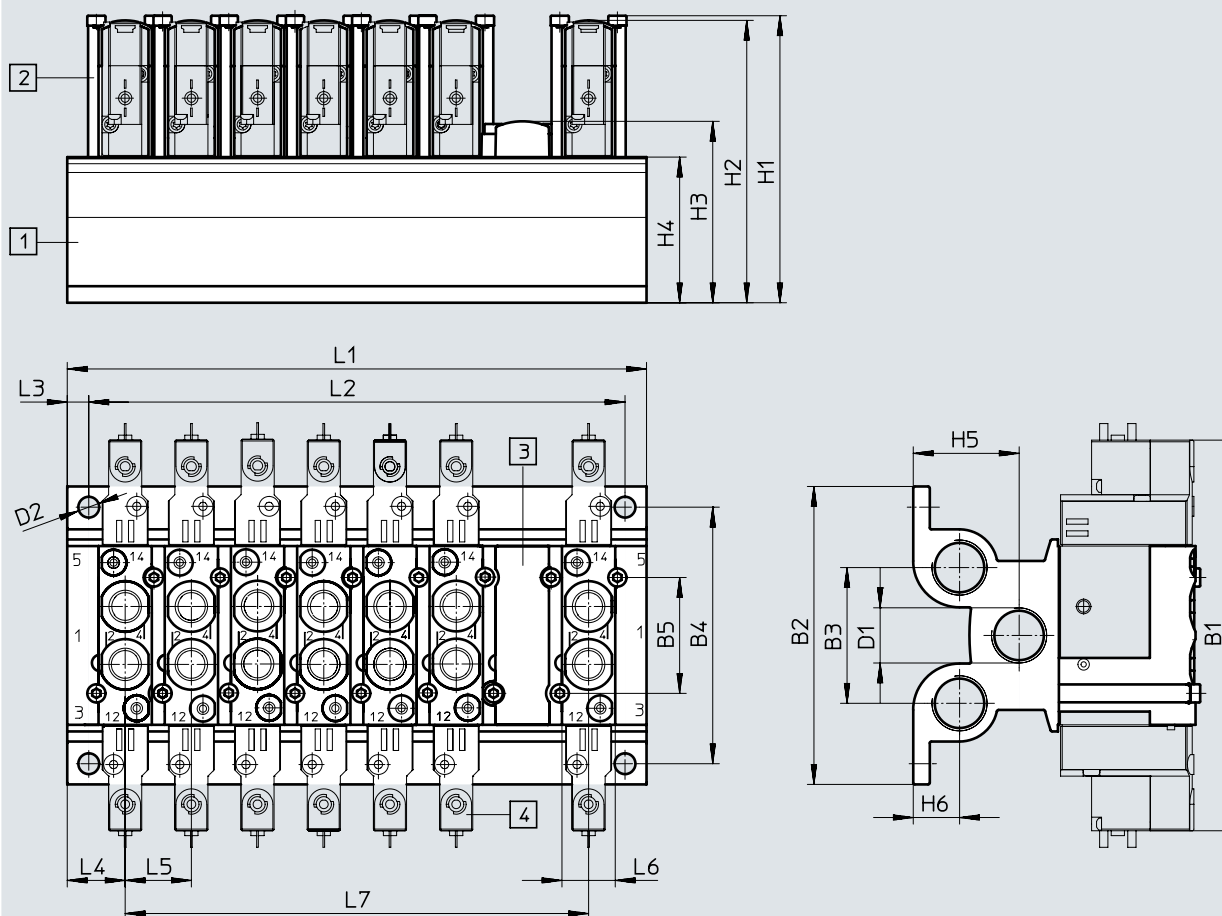
[1] přípojovací blok, rozteč 26 mm
